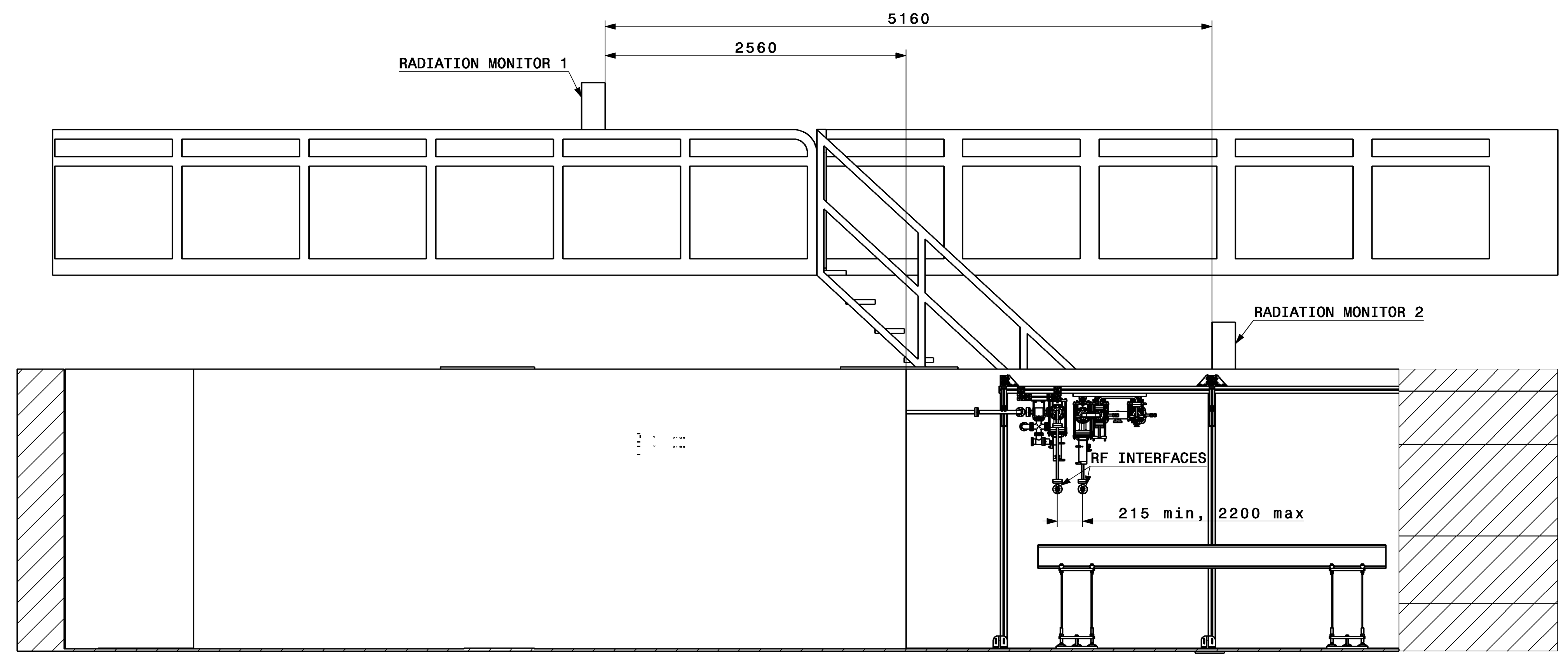
Section view B-B Scale: 1:25
