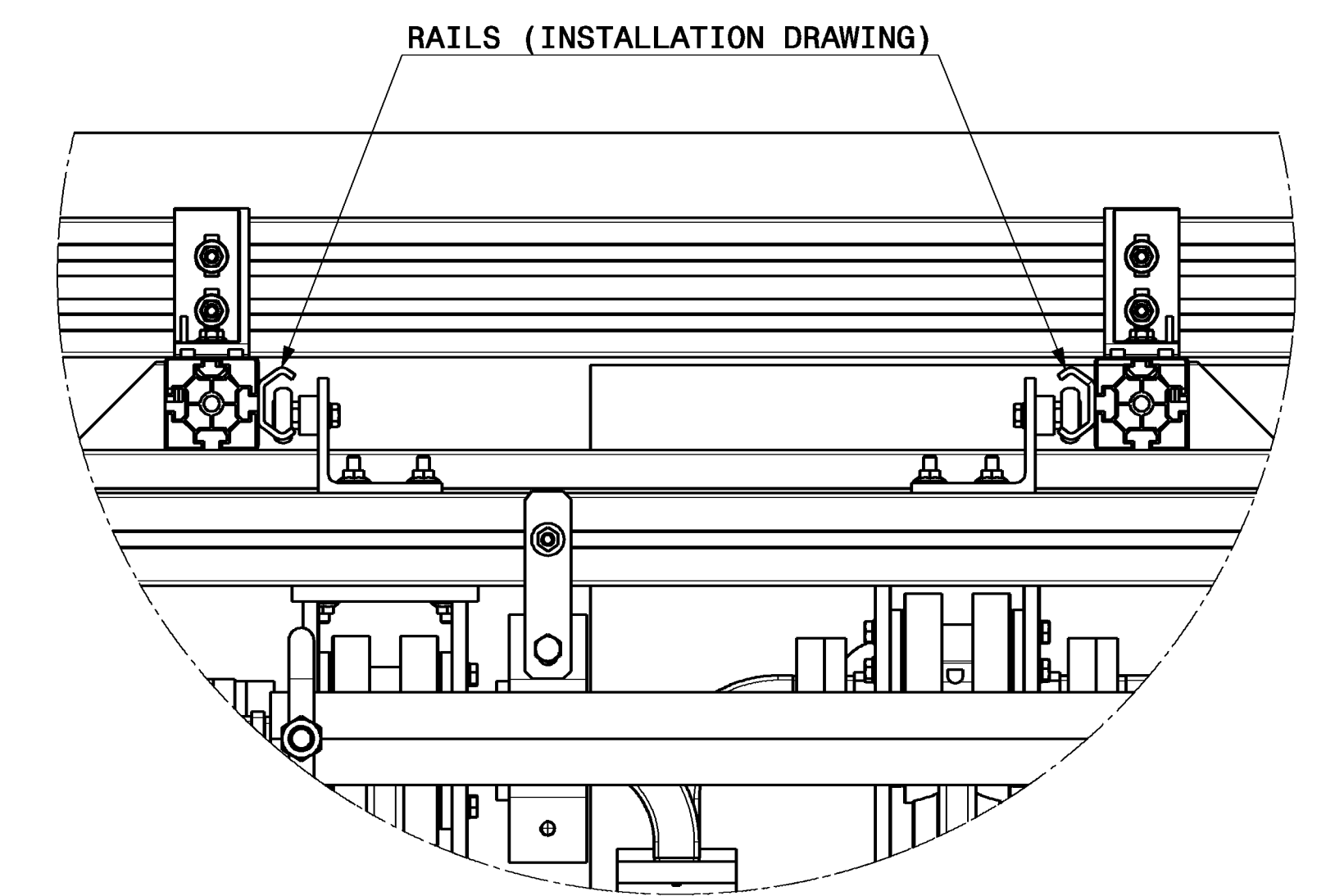
Detail C Scale: 1:4
