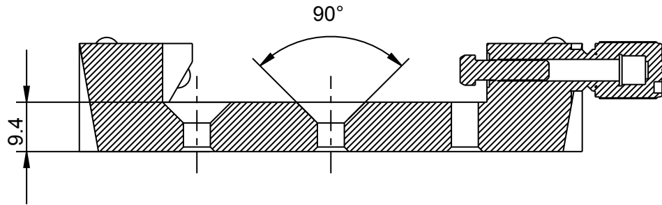
Detail A-A
